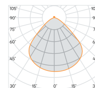
Г90 - глубокая 90°
